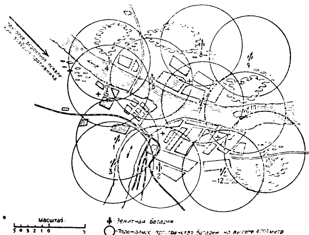
Черт. 3. Схема группового расположения зенитной артиллерии при обороне крупного центра.
